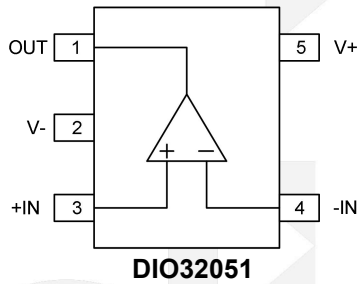
SOT23-5/SC70-5
