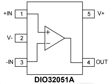
SOT23-5/SC70-5
