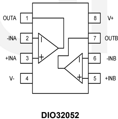
SOIC-8/MSOP-8/TSOT23-8
