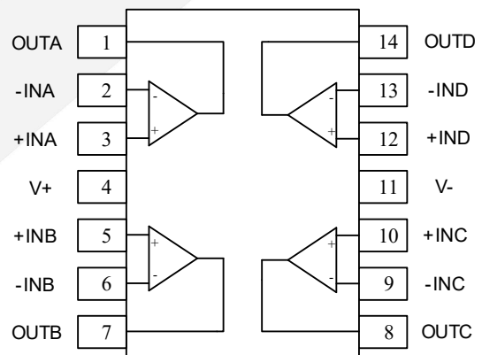
SOP-14/TSSOP-14
