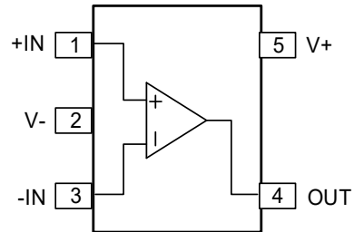
SOT23-5/SC70-5
