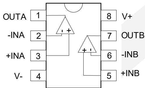
SOIC-8/MSOP-8
