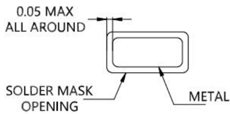
PADS 4-6 NON SOLDER MASK DEFINED
