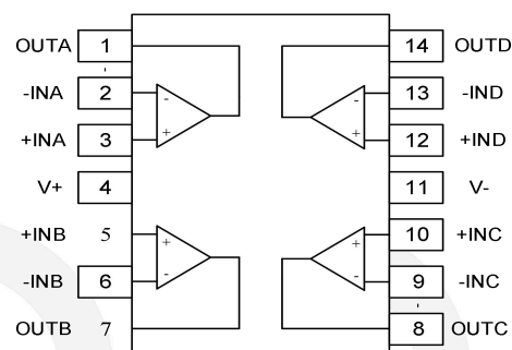
DIO29004 SOP-14/TSSOP-14
